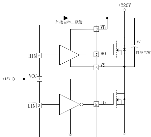
图 8-3. EG2131D 自举电路结构
