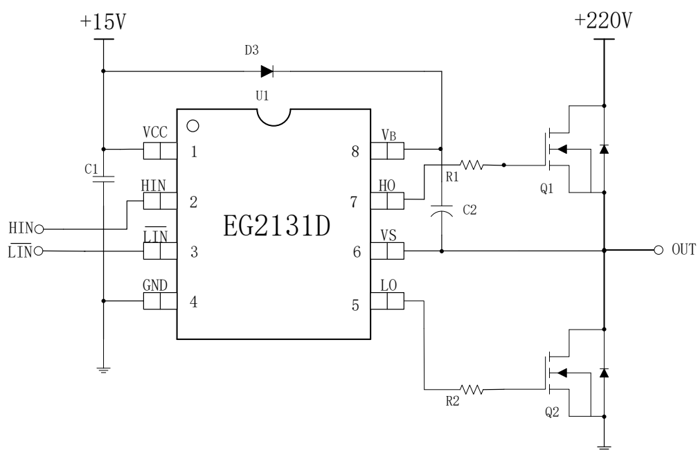
图 6-1. EG2131D 典型应用电路图
