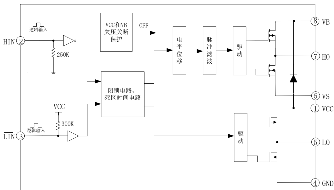
图 5-1. EG2131D 内部电路图
