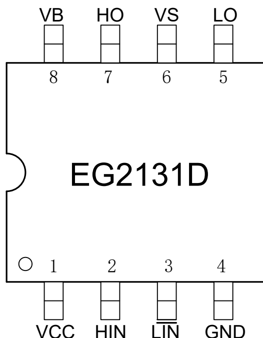
图 4-1. EG2131D 管脚定义
